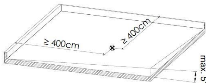
Kiesfangleiste
